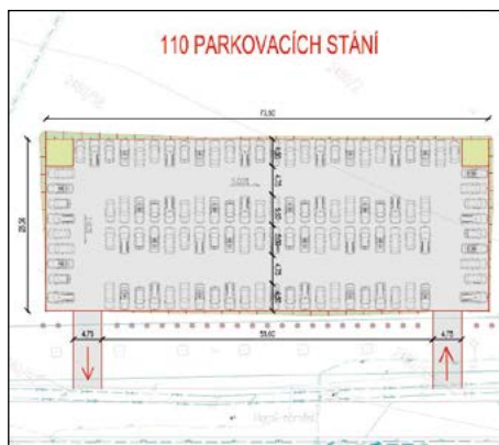
Situací výkres provizorního parkoviště
